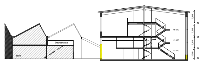
Schnitt
